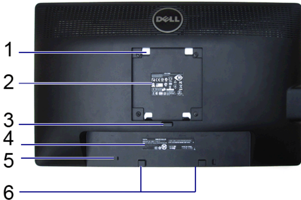
Vista trasera
